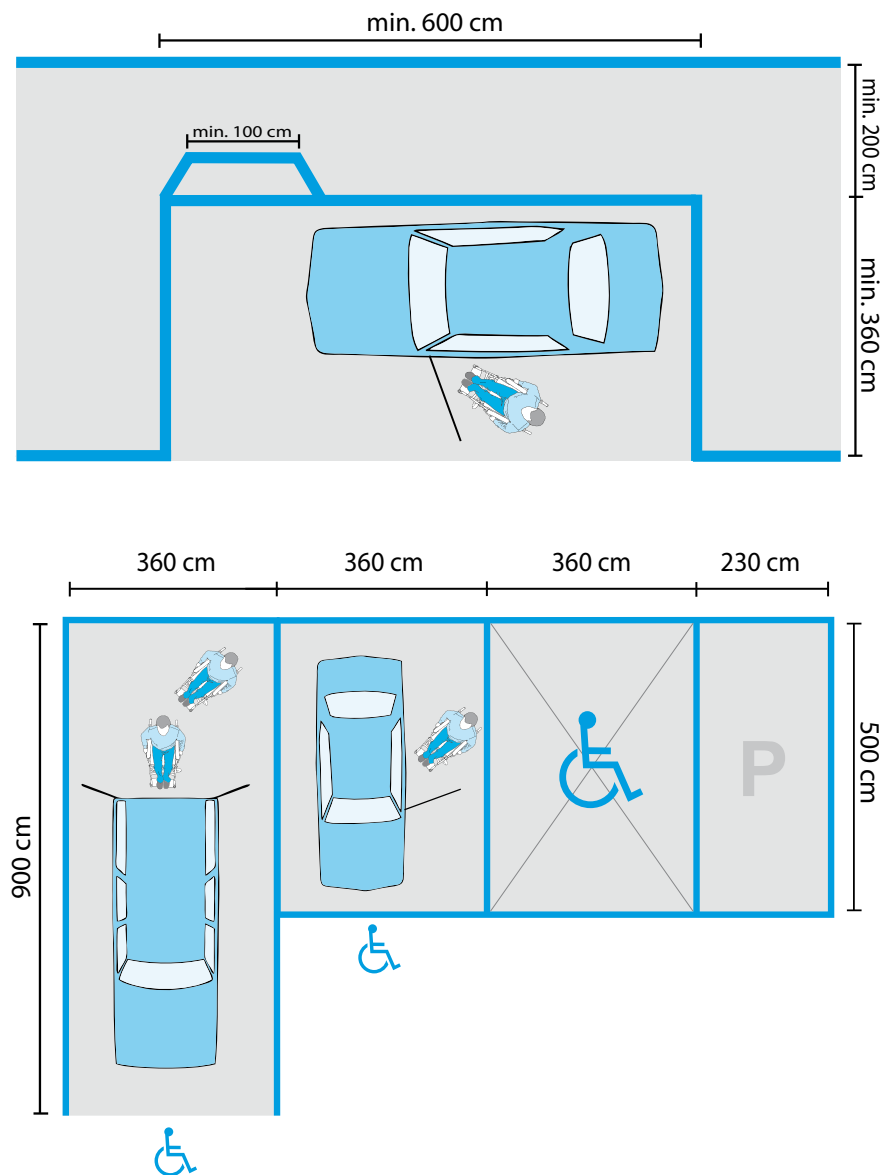
Rys. 75. Wymiary miejsc parkingowych.
