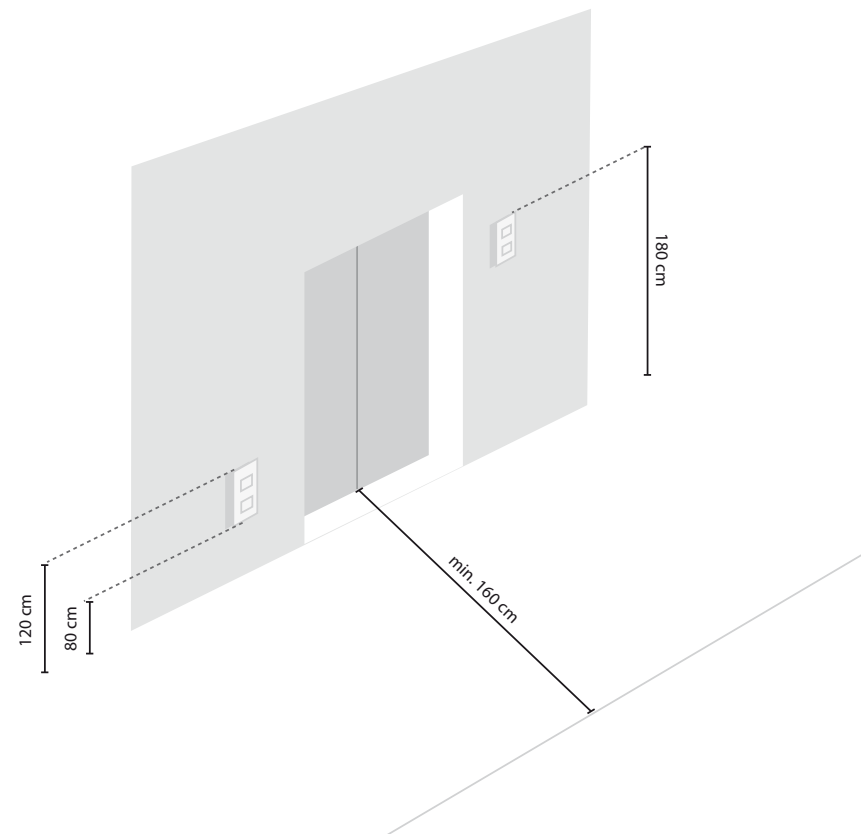
Rys. 24. Parametry przestrzeni przed wejściem do windy.
