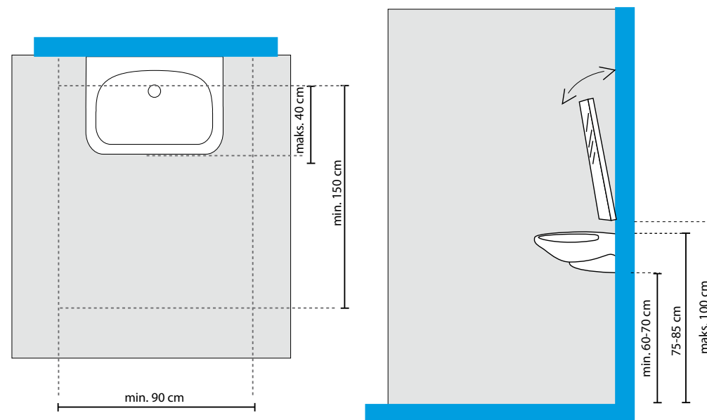
Rys. 65. Sposób montażu umywalki. Opracowanie własne, w oparciu o normę ISO 21542:2011.
