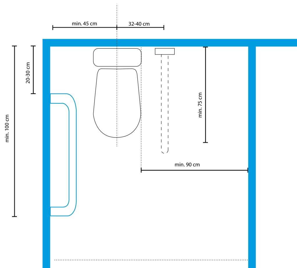
Rys. 63. Przykładowe położenie muszli ustępowej. Opracowanie własne, na podstawie normy ISO 21542:2011 oraz ADA.Standards for Accessible Design.
