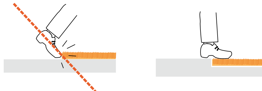
Rys. 34. Licowanie grubych chodników i wycieraczek z posadzką.
