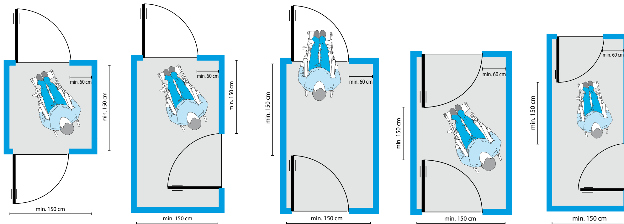
Rys. 46. Parametry przedsionków. Opracowanie własne, na podstawie normy ISO 21542:2011, pkt 10.8.2
