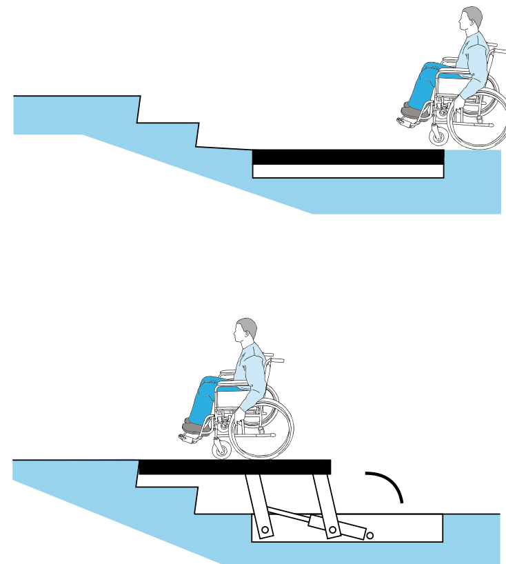
Rys. 30. Schematy działania innego rodzaju podnośników.
