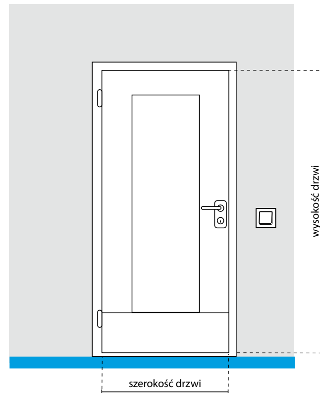
Rys. 42. Zasada pomiaru wielkości drzwi.
