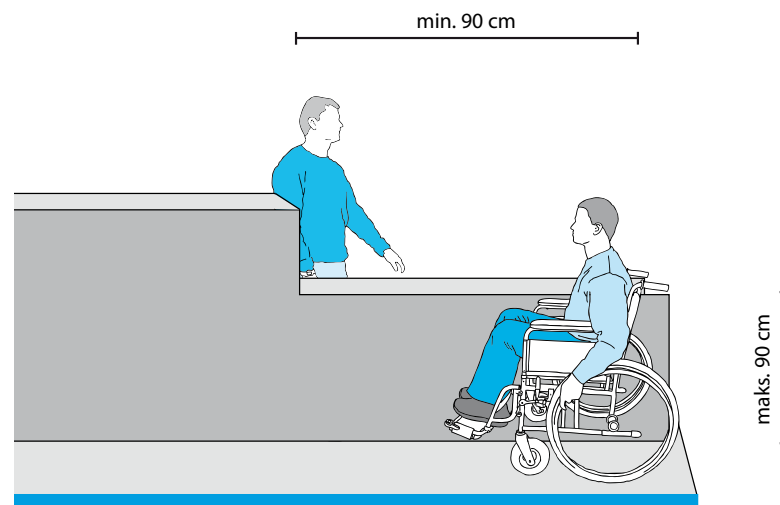
Rys. 73. Parametry blatu recepcji.
