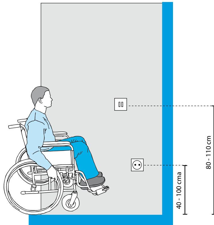
Rys. 79. Rozmieszczenie osprzętu elektrycznego. Opracowanie własne, w oparciu o normę ISO 21542:2011.
