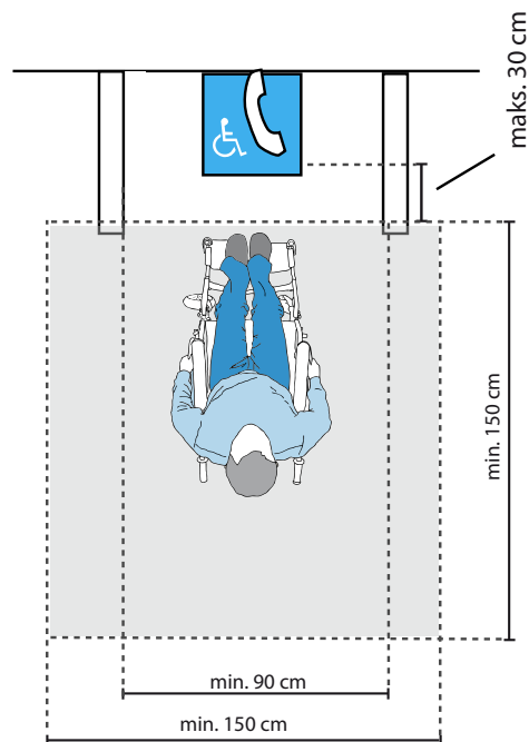
Rys. 57. Minimalna przestrzeń umożliwiającą osobie poruszającej się na wózku dotarcie do automatu telefonicznego.
