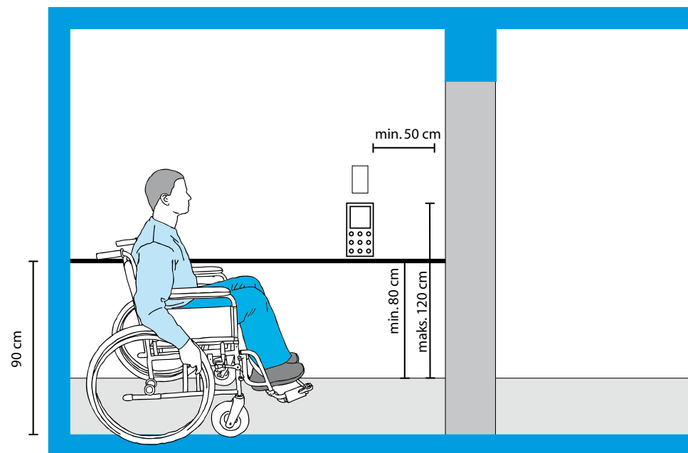
Rys. 25. Parametry wyposażenia kabiny dźwigu osobowego.
