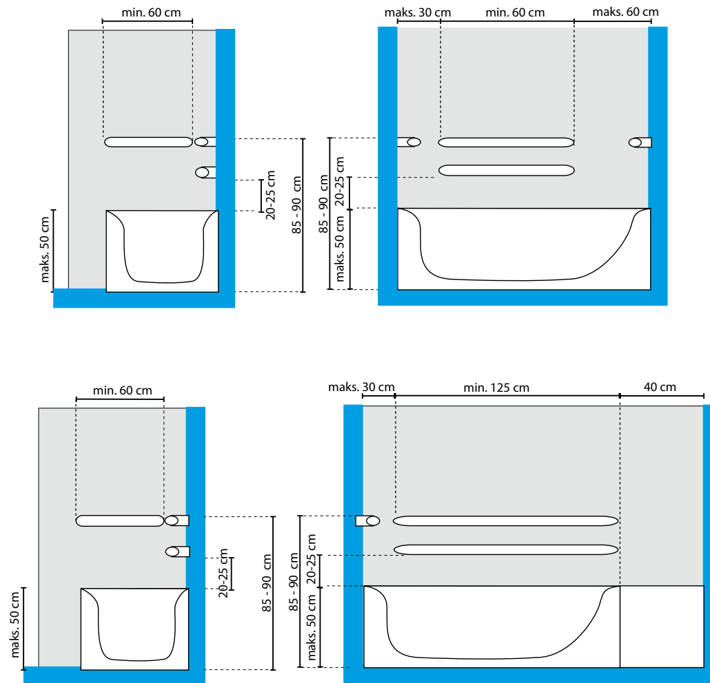
Rys. 67. Rozmieszczenie poręczy przy wannie. Opracowanie własne na podstawie ADA. Standards for Accessible Design.
