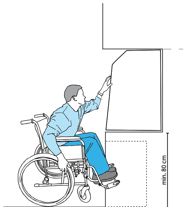
Rys. 60. Położenie elementów służących do obsługi automatu. Opracowanie własne, na podstawie normy ISO 21542:2011.
