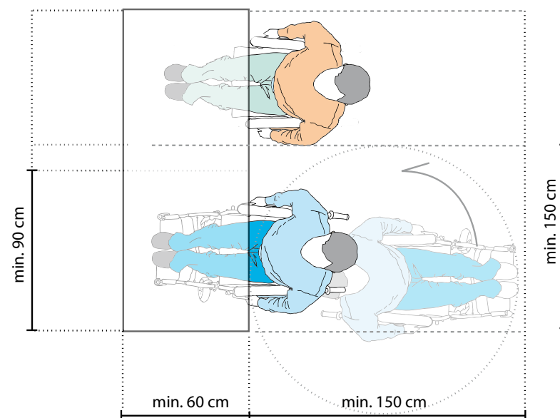
Rys. 54. Schemat miejsca przy stole, dostępnego dla osoby poruszającej się na wózku.
