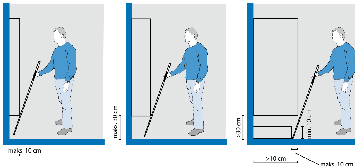
Rys. 51. Sposób projektowania wiszących przeszkód w sposób umożliwiający ich wykrycie przez osobę niewidomą. Opracowanie własne, na podstawie normy ISO 21542:2011, pkt. 7.14.
